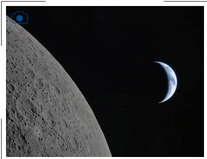
ثبت خورشیدگرفتگی از پشت ماه
